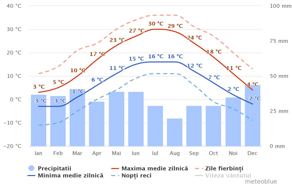
Figura Nr.5 – Temperatura și precipitațiile medii. Sursa: Meteoblue.com
