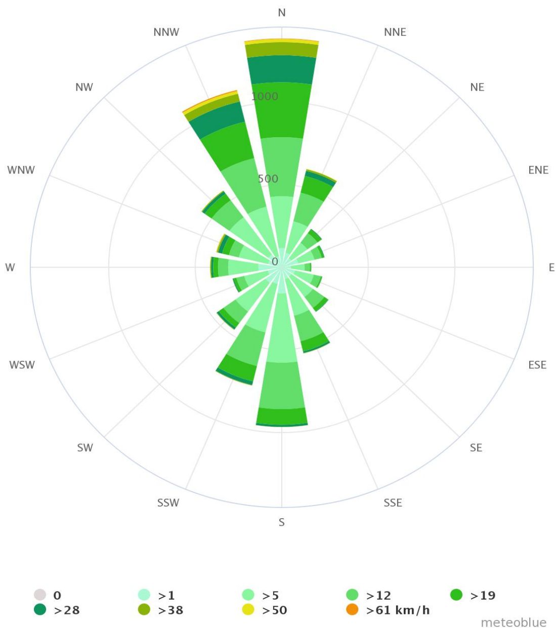
Figura Nr.10 – Roza vânturilor. Sursa: Meteoblue.com
