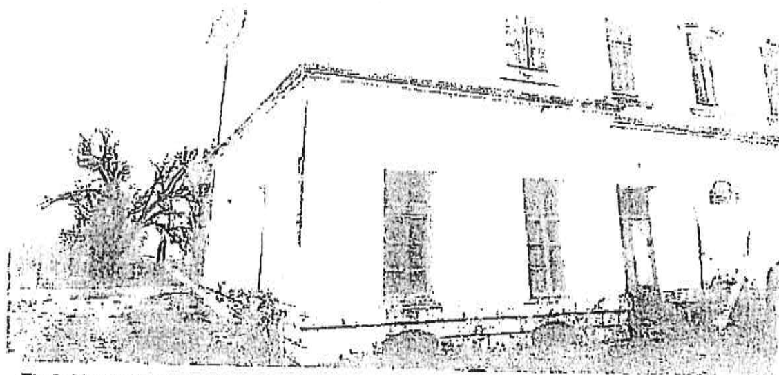
Fig.5: Lipsa trotuarelor perimetrare au permis apariția vegetației și stăgănca apelor la nivelul fundațiilor
