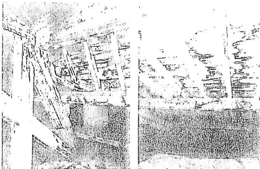
Fig. 11, 12: Infiltrații de apă la nivelul șarpantei existente
