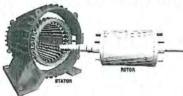
Figura 4.15. Componentele motorului electric asincron trifazat (Sursă: Learn Engineering).
