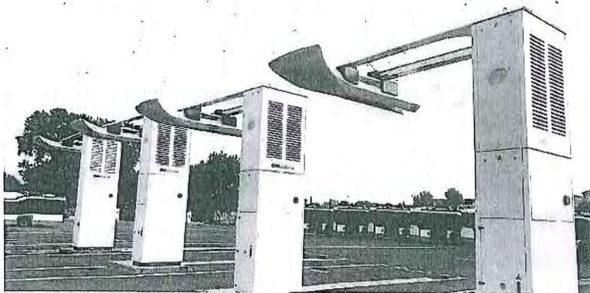
Figura 4.19. Infrastructură pentru încărcare rapidă, tip pantograph.
