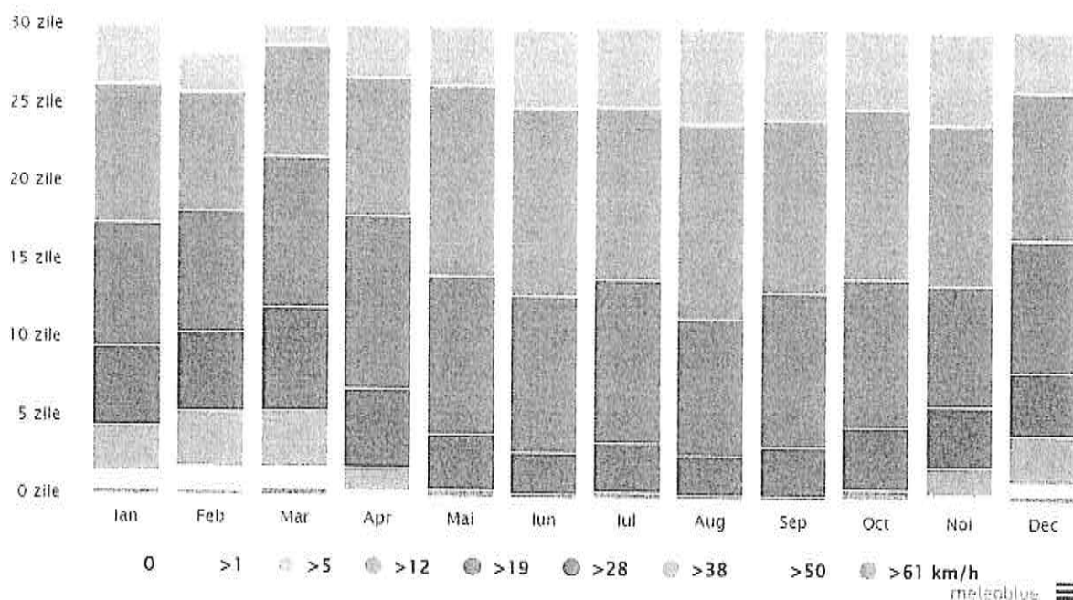
Fig. 8 – Viteza vântului
